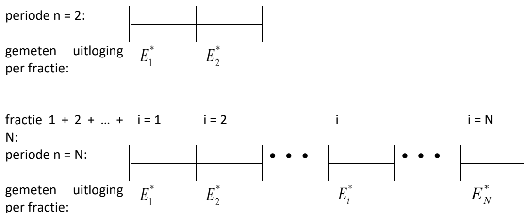
Figuur 1: Schematisch overzicht van termen die in deze norm worden gebruikt bij de bepaling van het uitlooggedrag van een proefstuk. De fracties i = 1 tot en met i = N duiden de opeenvolgende eluaatfracties aan; de periode n = x komt overeen met de som van het aantal fracties i = 1 tot en met i = x
