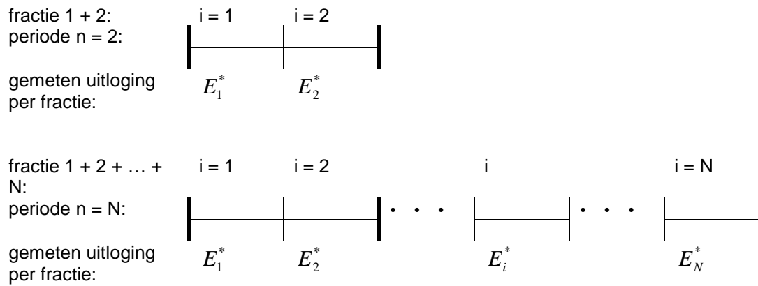
Figuur 1: Schematisch overzicht van termen die in deze norm worden gebruikt bij de bepaling van het uitlooggedrag van een proefstuk. De fracties i = 1 tot en met i = N duiden de opeenvolgende eluafracties aan; de periode n = x komt overeen met de som van het aantal fracties i = 1 tot en met i = x
