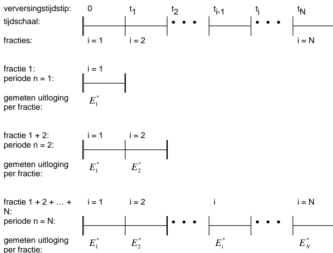
Figuur 1: Schematisch overzicht van termen die in deze norm worden gebruikt bij de bepaling van het uitlooggedrag van een proefstuk. De fracties i = 1 tot en met i = N duiden de opeenvolgende eluaatfracties aan; de periode n = x komt overeen met de som van het aantal fracties i = 1 tot en met i = x
