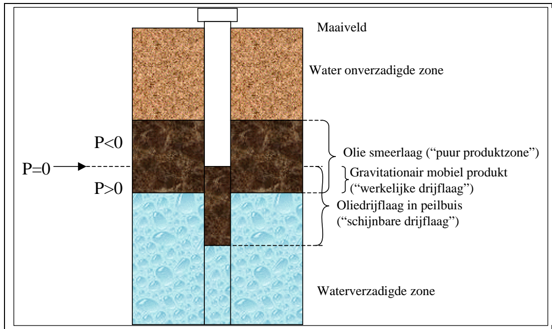
Figuur 4 - Schematische voorstelling van de wijze van voorkomen van een puur-productzone (olie) rond het grondwater niveau en de begrippen "schijnbare" en "werkelijke" drijf laag ( P = olie - capillaire druk, P = 0 : oliespiegel)
