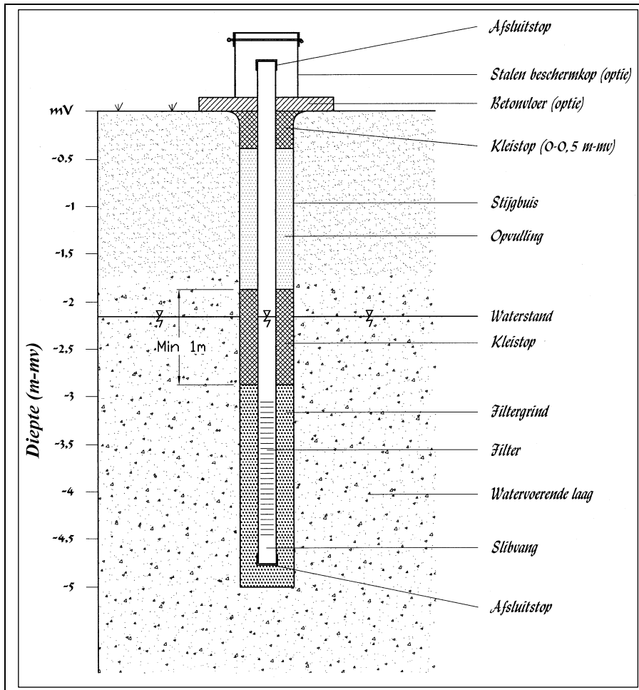
Figuur 2 – Schematische doorsnede van een boorgat met 1 peilbuis
