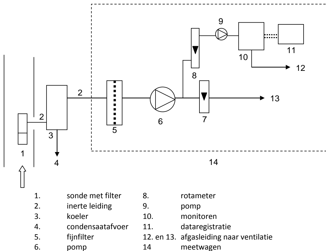
Figuur 2: Bemonstering van rookgassen met monitoren in een meetwagen
