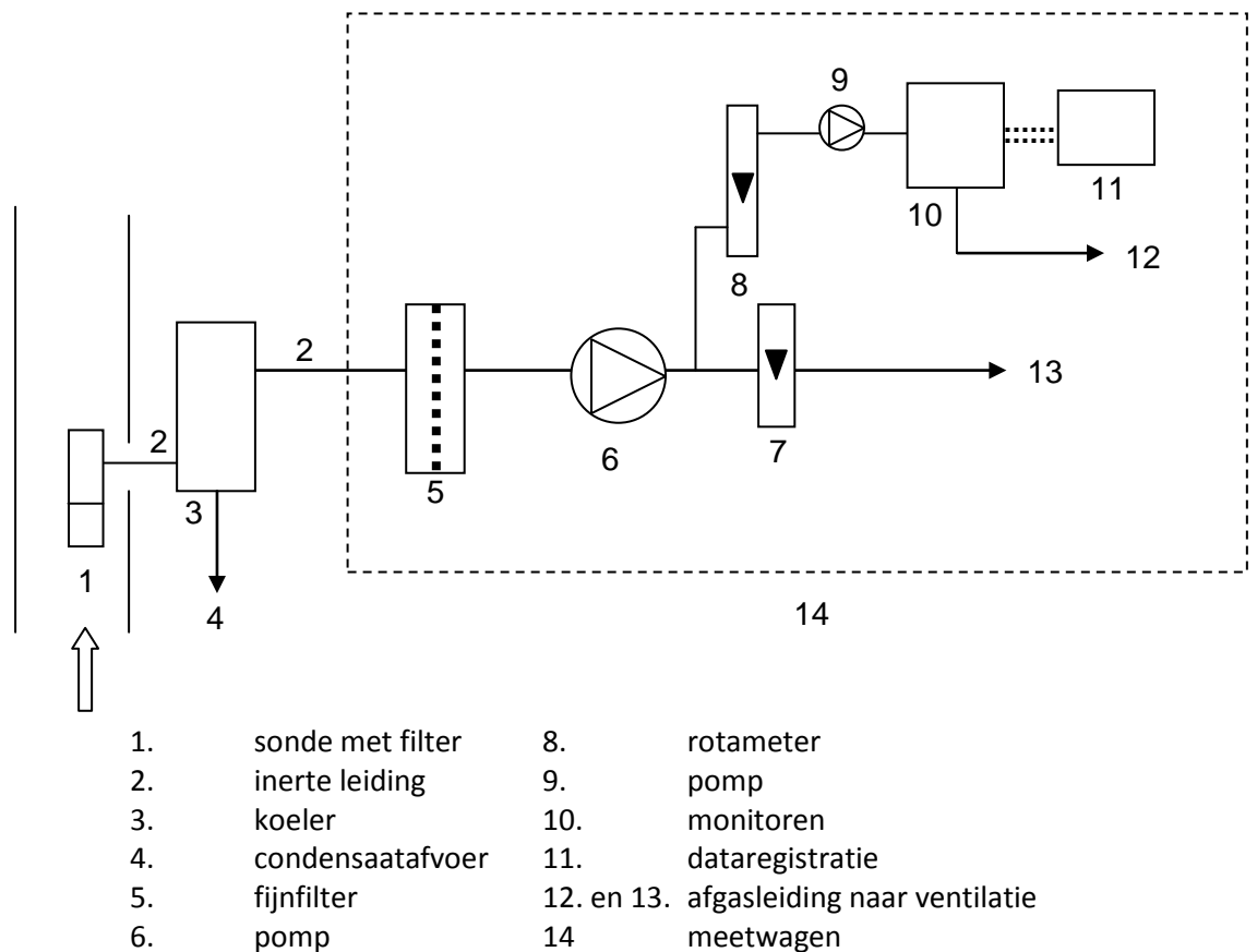
Figuur 2: Bemonstering van rookgassen met monitoren in een meetwagen
