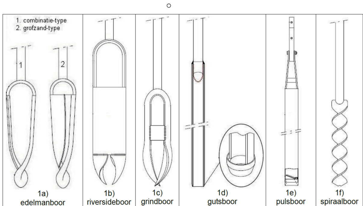
Figuur 1: Overzicht van verschillende handboren met de onverzadigde zone als voornaamste toepassingsgebied
