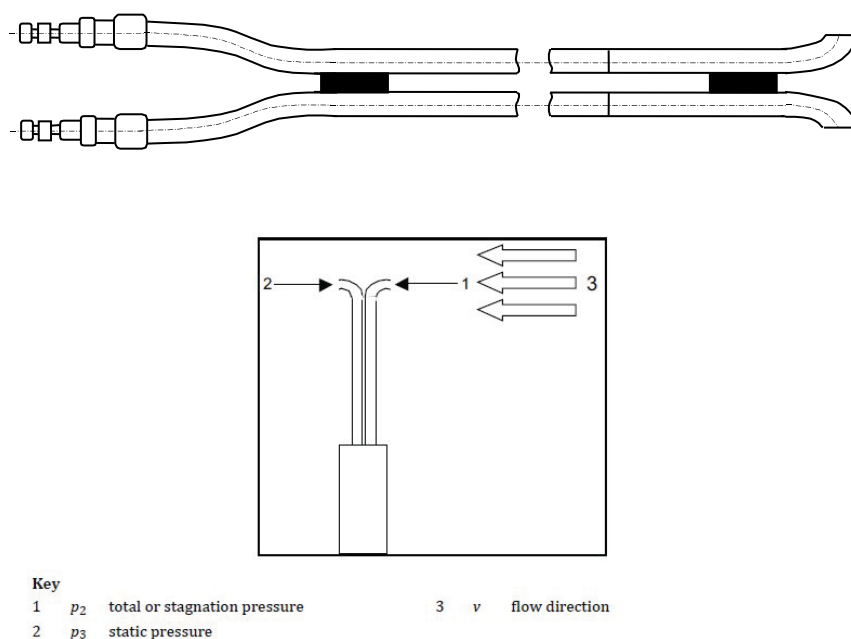
Figuur 3: S-type Pitotbuis en oriëntering in de gasstroom
