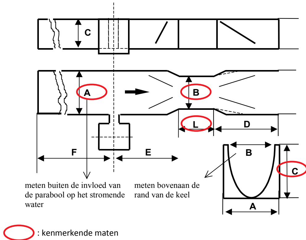
Figuur 2 Schematische voorstelling van meetgoot met parabolische bodem met aanduiding van maten
