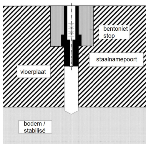
Figuur 7: Sub-slab staalnamesysteem (WDNR, 2014)
