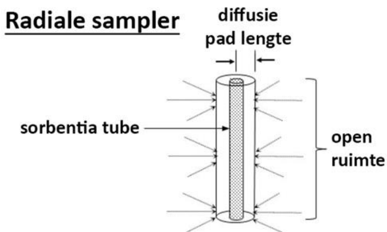
Figuur 2: Overzicht passieve diffusiegebaseerde luchtsamplers (Dowson et al., 2015)
