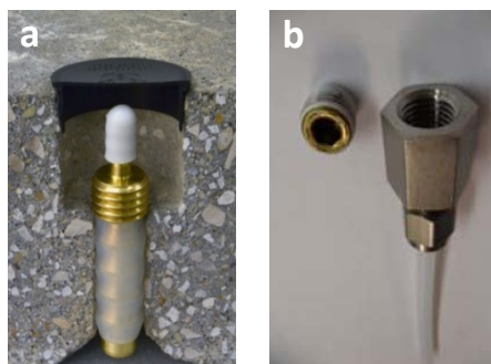
Figuur 6: Sub-slab staalnamesysteem (HEER, 2014)
