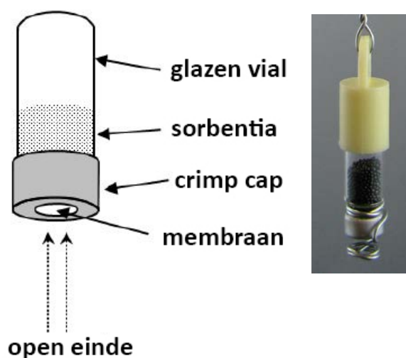
Figuur 3: Passieve permeatiegebaseerde luchtsampler
