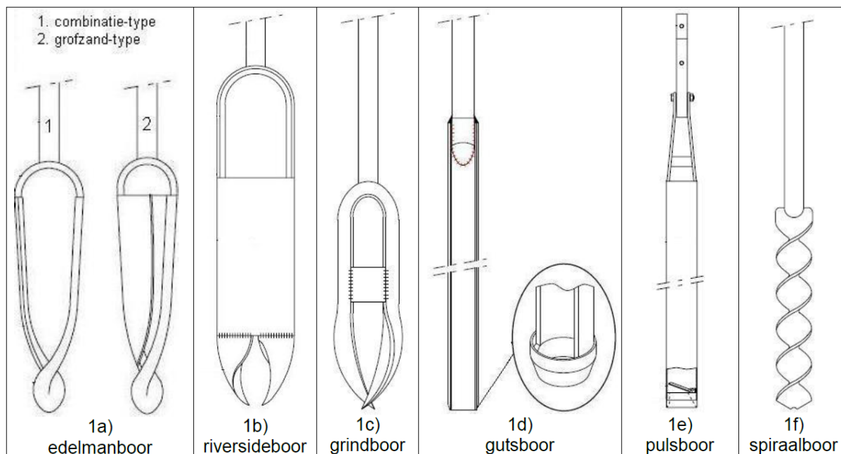
Figuur 1: Overzicht van verschillende handboren met de onverzadigde zone als voornaamste toepassingsgebied
