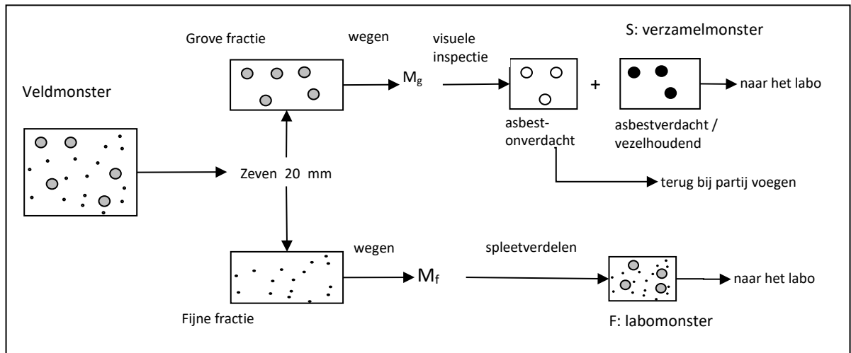
Figuur 2 : schema monstervoorbehandeling
