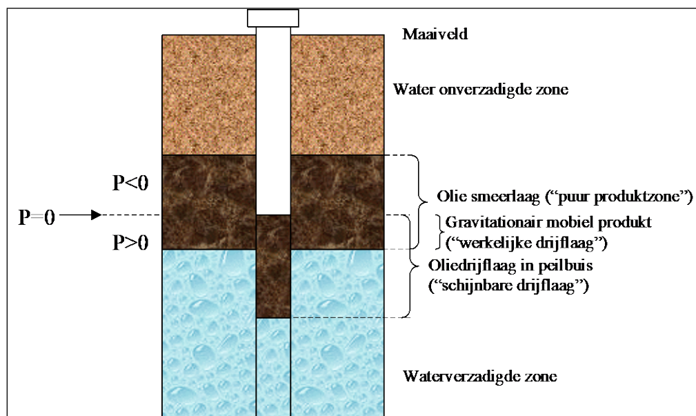
Figuur 5 - Schematische voorstelling van de wijze van voorkomen van een puur-productzone (olie) rond het grondwaterniveau en de begrippen "schijnbare" en "werkelijke" drijfslag ( P = olie - capillaire druk, P = 0 : oliespiegel)
