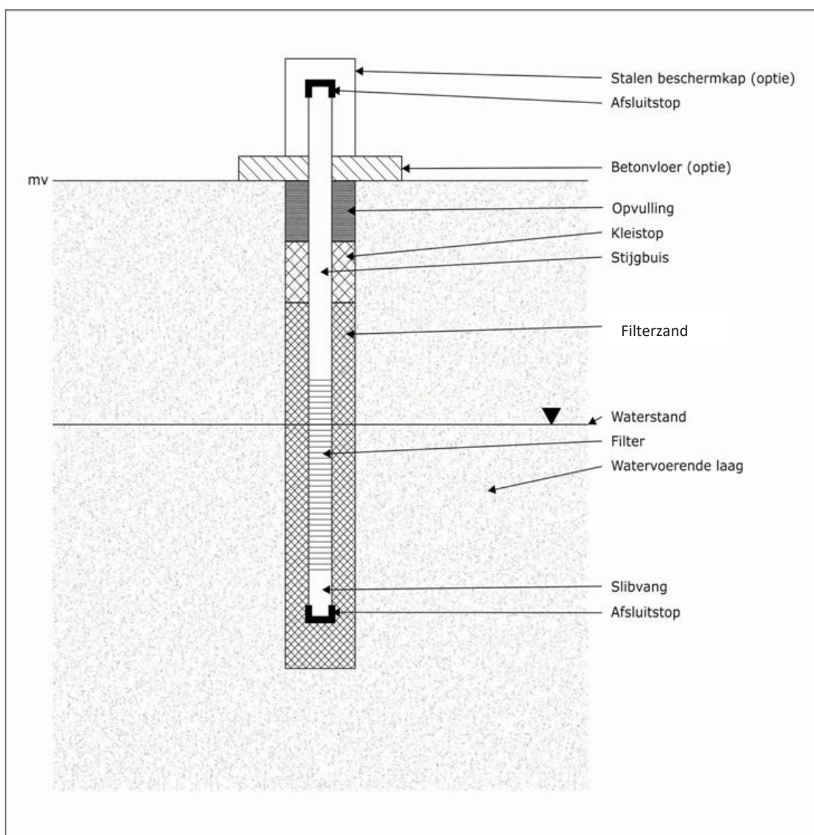
Figuur 1: schematische doorsnede van een boorgat met snijdende peilbuis (bron: CMA/1/A.2)
