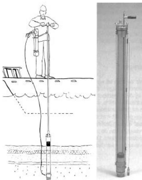
Figuur 3: Beekersampler
