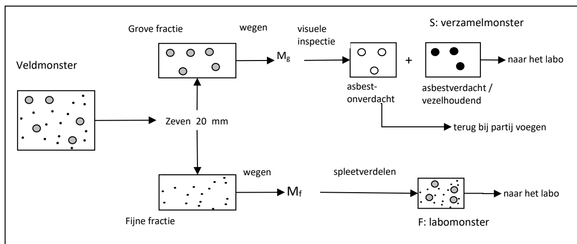
Figuur 2 : schema monsterveroorbehandling
