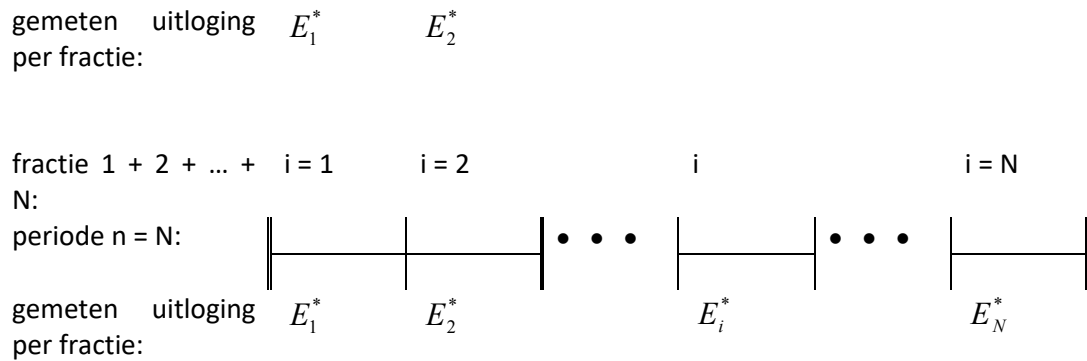
Figuur 1: Schematisch overzicht van termen die in deze norm worden gebruikt bij de bepaling van het uitloggedrag van een proefstuk. De fracties i = 1 tot en met i = N duiden de opeenvolgende eluaatfracties aan; de periode n = x komt overeen met de som van het aantal fracties i = 1 tot en met i = x
