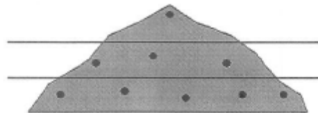
Figuur 3: verdeling van bemonsteringsplaatsen in een voorraadhoop (zij aanzicht)
