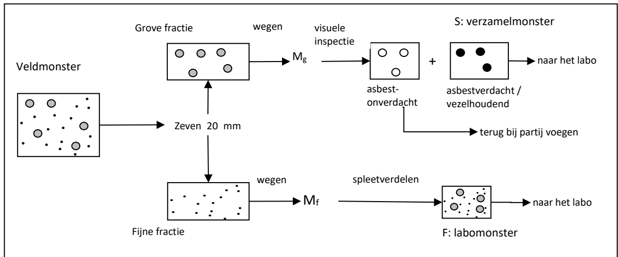
Figuur 2 : schema monsterveroорbehandling
