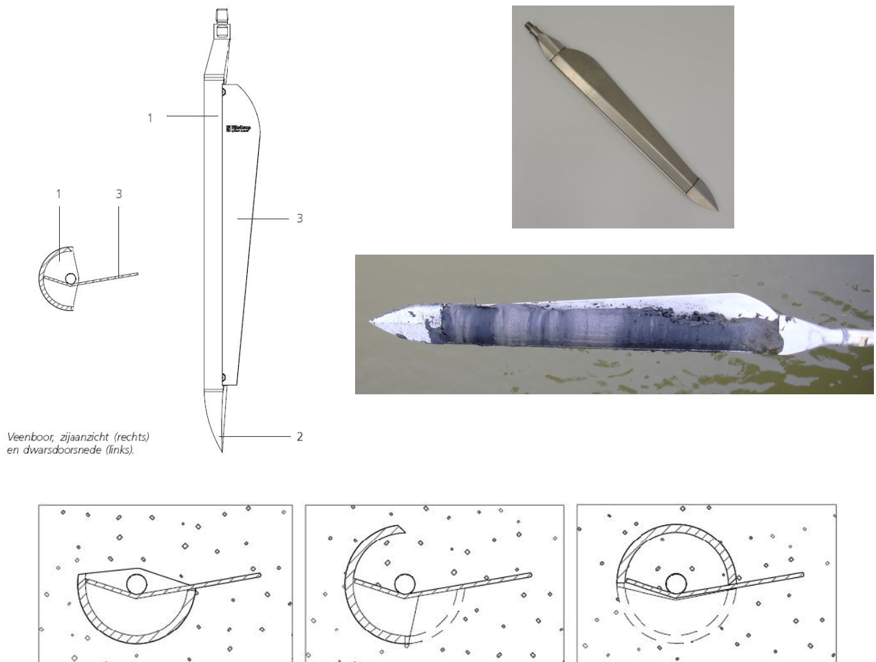
Figuur 2: Veenboor
