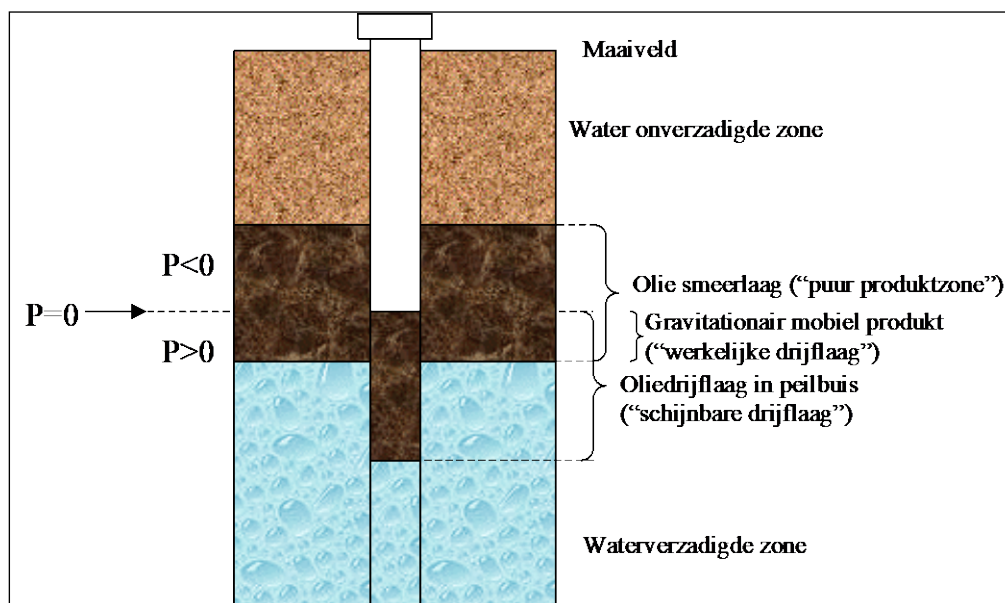
Figuur 5 - Schematische voorstelling van de wijze van voorkomen van een puur-productzone (olie) rond het grondwatervniveau en de begrippen “schijnbare” en “werkelijke” drijfslaag ( P = olie - capillaire druk, P = 0 : oliespiegel)
