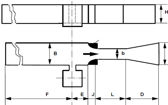
Meetgoot met vlakke bodem: maten
