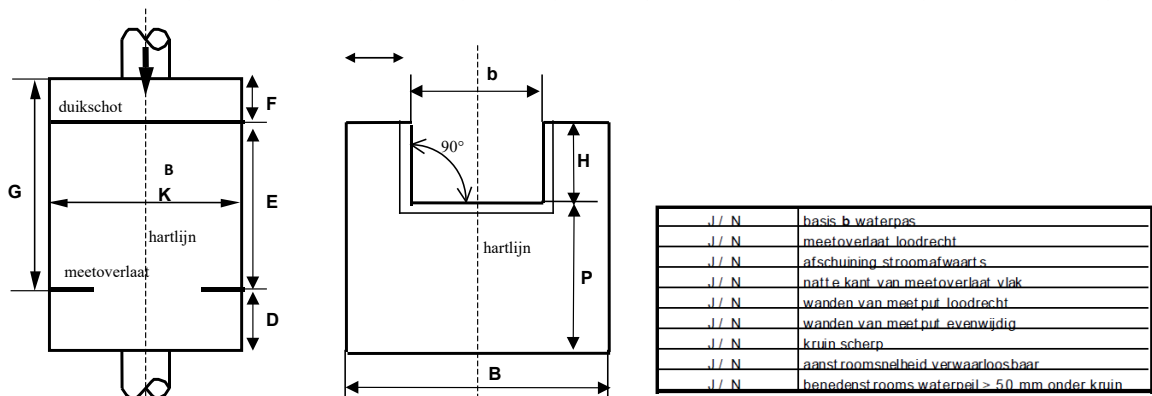
Rechthoekig meetschot met contractie: maten
