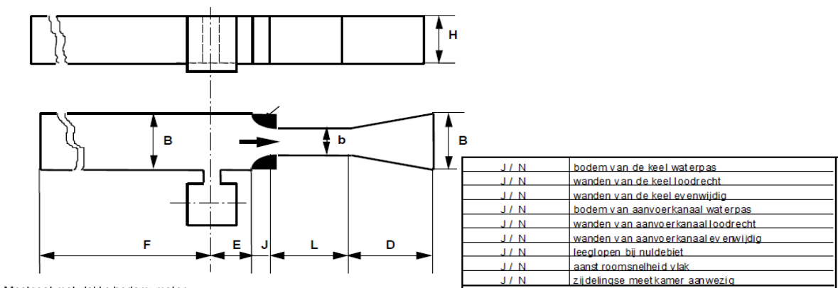
Meetgoot met vlakke bodem: maten
