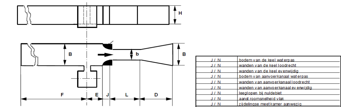
Meetgoot met vlakke bodem: maten
