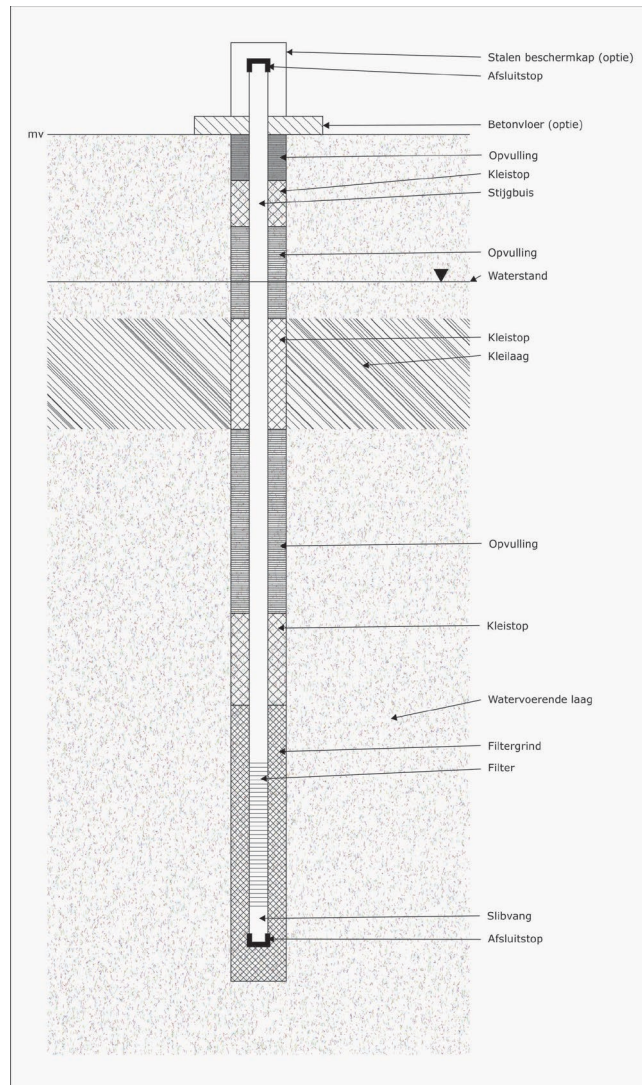
Figuur 3 – Schematische doorsnede van een boorgat met een peilbuis waarvan de filter is gelegen onder een slecht doorlatende laag (niet op schaal)
