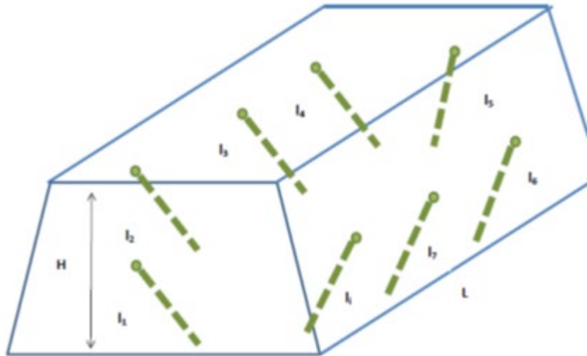
Figuur 2: Verdeling van ondiepe boringen langs de omtrek van één (virtuele deel)partij: l_1+l_2+l_3+l_4+l_5+l_6+l_7+l_i \geq 1.5 \times \text{langste zijde (L of B of H)}
