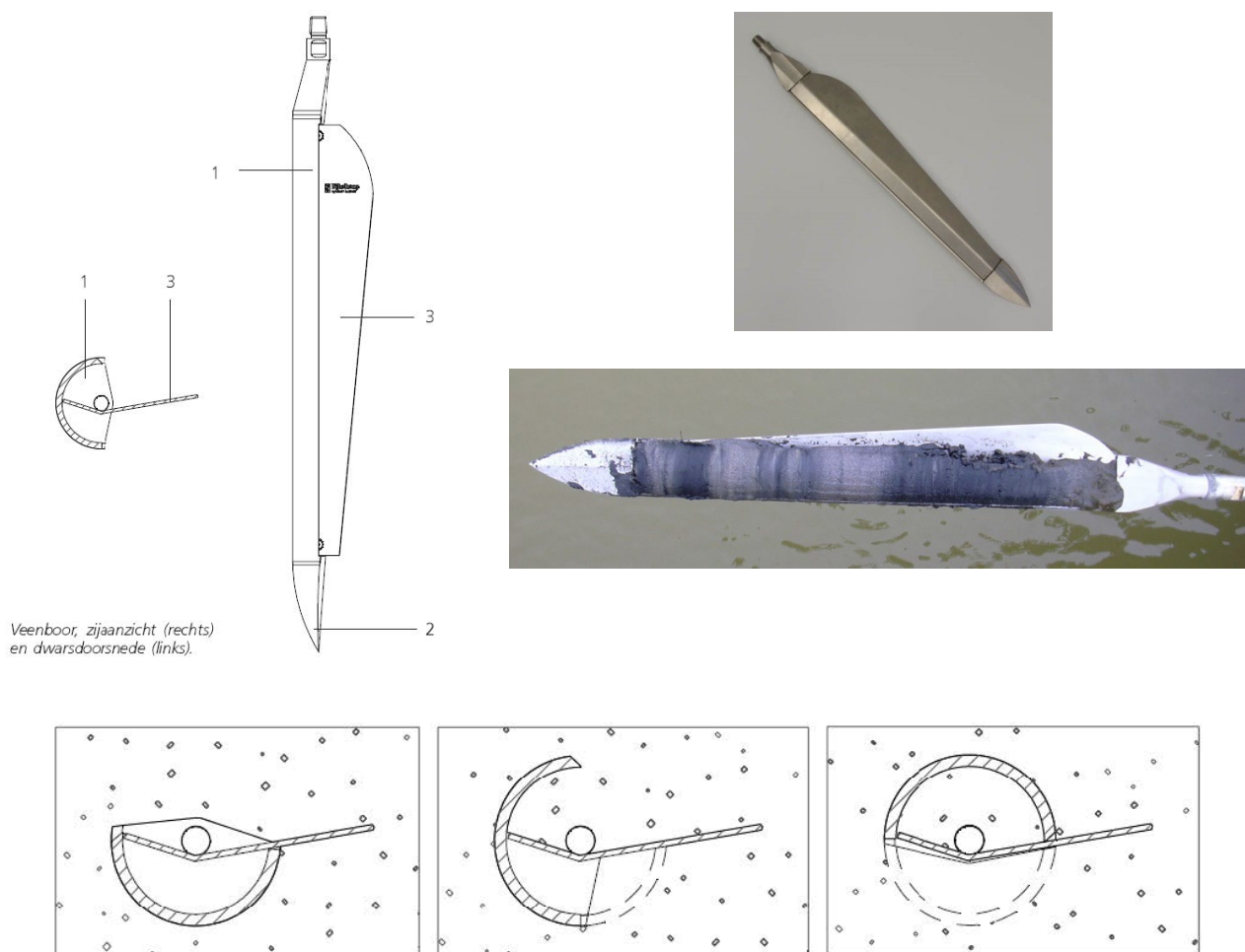
Figuur 2: Veenboor
