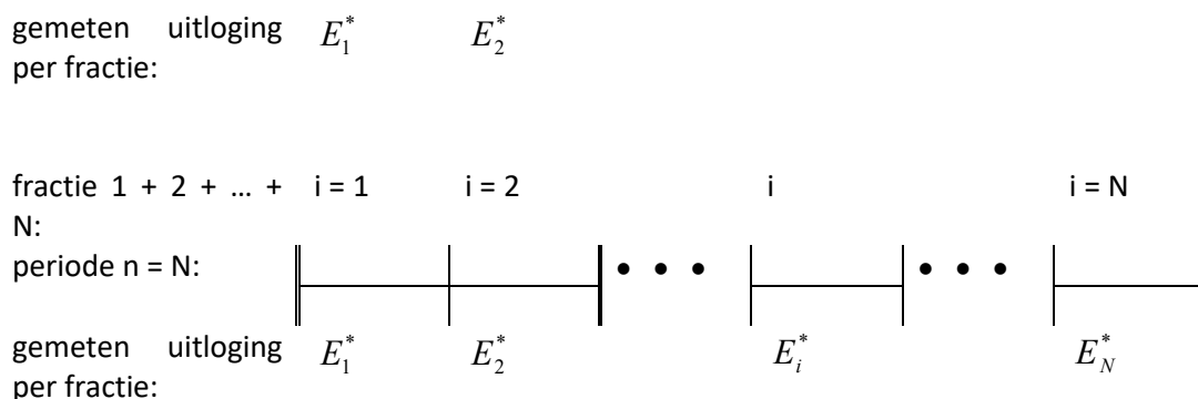
Figuur 1: Schematisch overzicht van termen die in deze norm worden gebruikt bij de bepaling van het uitlooggedrag van een proefstuk. De fracties i = 1 tot en met i = N duiden de opeenvolgende eluatfracties aan; de periode n = x komt overeen met de som van het aantal fracties i = 1 tot en met i = x
