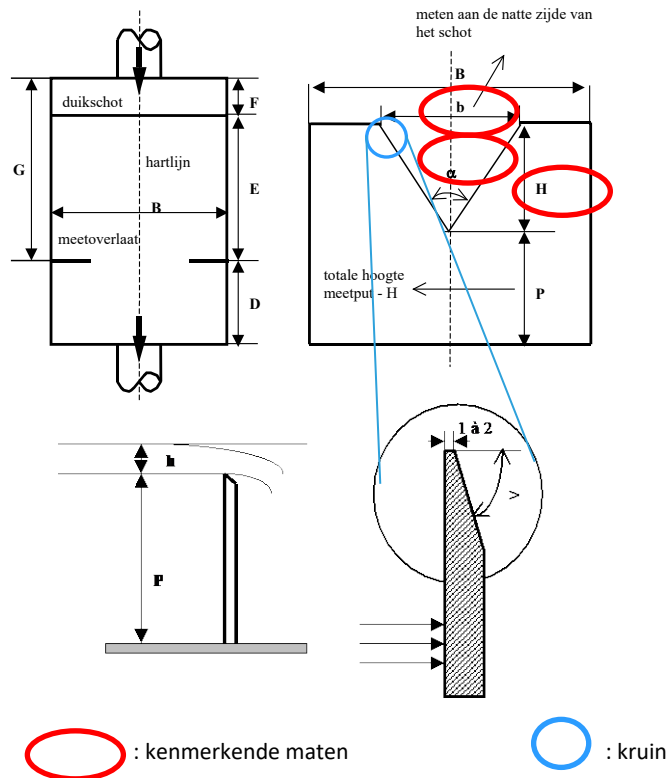
Figuur 6: Schematische voorstelling van meetschot met Thomson overlaat met aanduiding van maten (bron: VMM) [B: breedte van het aanvoer kanaal; \alpha : hoek van de V-vormige uitsnijding; H: hoogte van de V-vormige uitsnijding; h: waterhoogte; P: hoogte van het puntje van de V-vormige uitsnijding ten opzichte van de vloer; D: stroomafwaartse afstand van het meetschot tot aan de putwand; E: afstand tussen duikschot en meetschot; F: stroomopwaartse afstand van putwand tot aan het duikschot; G: stroomopwaartse afstand van de putwand tot aan het meetschot]
