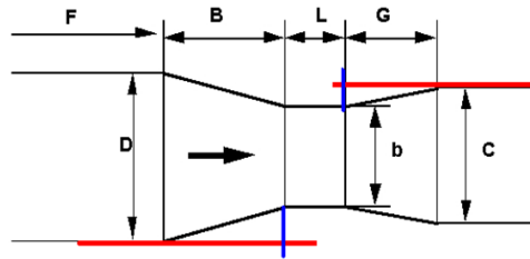
Figuur 8: Opmeting B en G bij type Parshall [bron: VMM]
