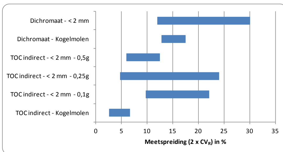
Figuur 22 Inschatting totale meetspreiding (95% B.I.) bij de bepaling van het organische koolstofgehalte in bodem ifv analysetechniek, monstervoorbehandeling en testportie
