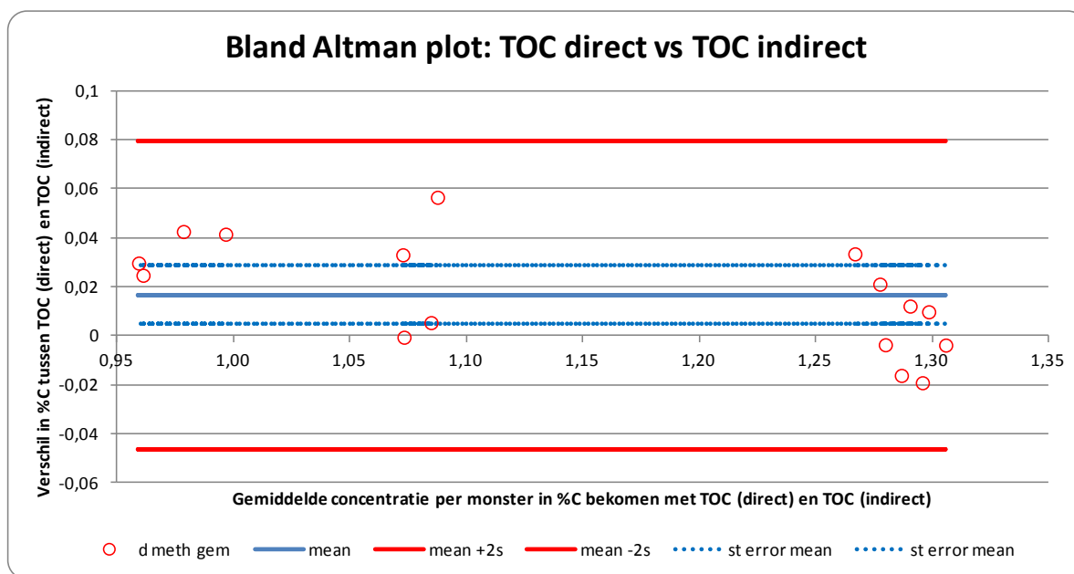
Figuur 18 Bland Altman plot van het absoluut verschil tov het gemiddelde voor de bepaling van TOC met de directe en de indirecte methode
