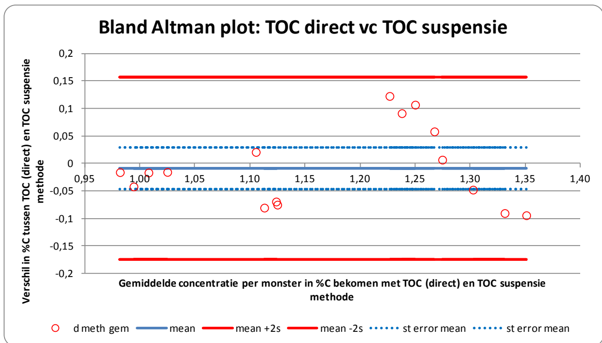
Figuur 19 Bland Altman plot van het absoluut verschil tov het gemiddelde voor de bepaling van TOC met de directe en de suspensie methode
