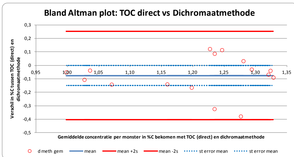
Figuur 20 Bland Altman plot van het absoluut verschil tov het gemiddelde voor de bepaling van TOC met de directe methode en de dichromaatmethode
