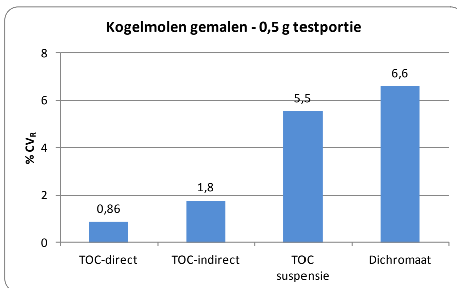
Figuur 17 Analytische meetspreiding van gehalte organische koolstof ifv de methode
