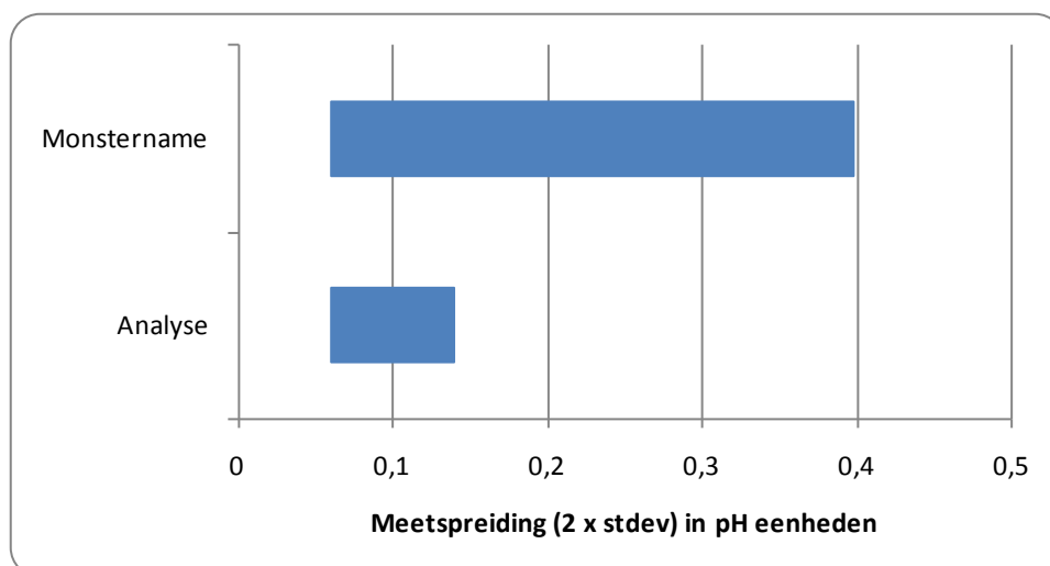
Figuur 21 Inschatting meetspreiding (95% B.I.) bij de bepaling van pH in bodem
