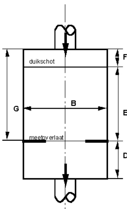
Figuur 6: schematische voorstelling van de constructie van een meetput voor meetschotten [B: breedte van het aanvoerkanal; D: stroomafwaartse afstand van het meetschot tot aan de putwand; E: afstand tussen duikschot en meetschot; F: stroomopwaartse afstand van putwand tot aan het duikschot; G: stroomopwaartse afstand van de putwand tot aan het meetschot] (bron: VMM)
