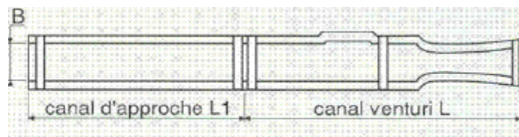
Figuur 9: Schematische voorstelling van meetgoot type Hydrologic serie 1253 met aanduiding van maten (bron: Elscolab ® ) [B: breedte van het aanvoerkanaal; L1: lengte van het aanvoerkanaal; L: lengte meetsectie; F: lengte aanvoerkanaal-hartlijn meetput; H: hoogte van de meetgoot]
