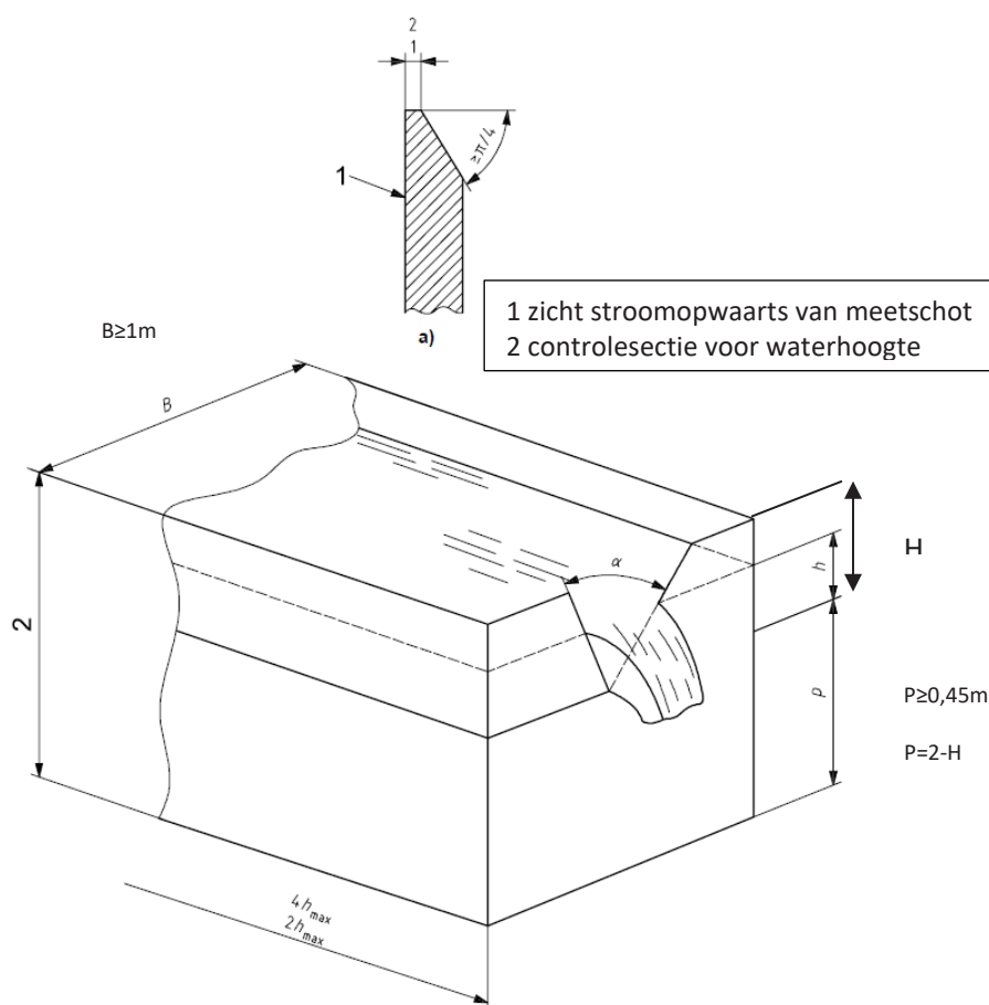
Figuur 5: geometrie van een V-schot (bron ISO 1438:2008)
