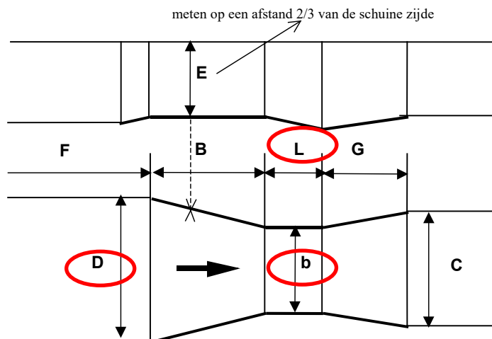
Figuur 11: Schematische voorstelling van Venturi meetgoot type Parshall met aanduiding van maten (bron: VMM) [ b : breedte van de vernauwing; B : lengte van het convergerende gedeelte voor de vernauwing; C : breedte van het afvoerkanaal; D : breedte van het aanvoerkanaal; E : afstand van de verhoging tot de rand van de meetgoot; L : lengte van de vernauwing; G : lengte van het divergerende gedeelte na de vernauwing]
