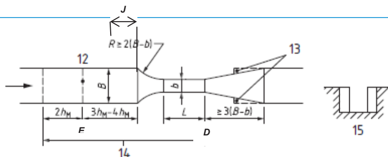
Figuur 4: geometrie van een meetgoot met vlakke bodem, rechthoekige doorsnede en lange keel [1: verbindingkanaal meetput; 2: meetput; 3: aanvoerkanaal; 4: convergerende zone R (ingang meetsectie); 5: keel; 6: divergerende zone D (uitgang meetsectie); 7: afkapping divergerende zone (niet bij standaard meetgoten); 8: opwaartse golfbeweging; 9: afvoerkanaal; 10: zijdelings insprong wanden; 11: stroomrichting; 12: controlesectie voor waterhoogte; 13: de divergerende zone kan ook afgekapt worden op halve lengte indien de recovery van de waterhoogte in het uitvoerkanaal niet belangrijk is; 14: in een meetgoot met vlakke bodem moeten aanvoerkanaal en keel horizontaal waterpas liggen over de volledige lengte en breedte.] (bron: ISO 4359:2013)
