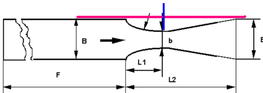
Figuur 8: Opmeting L1 en L2 bij Venturi type Khafagi (bron: VMM)
