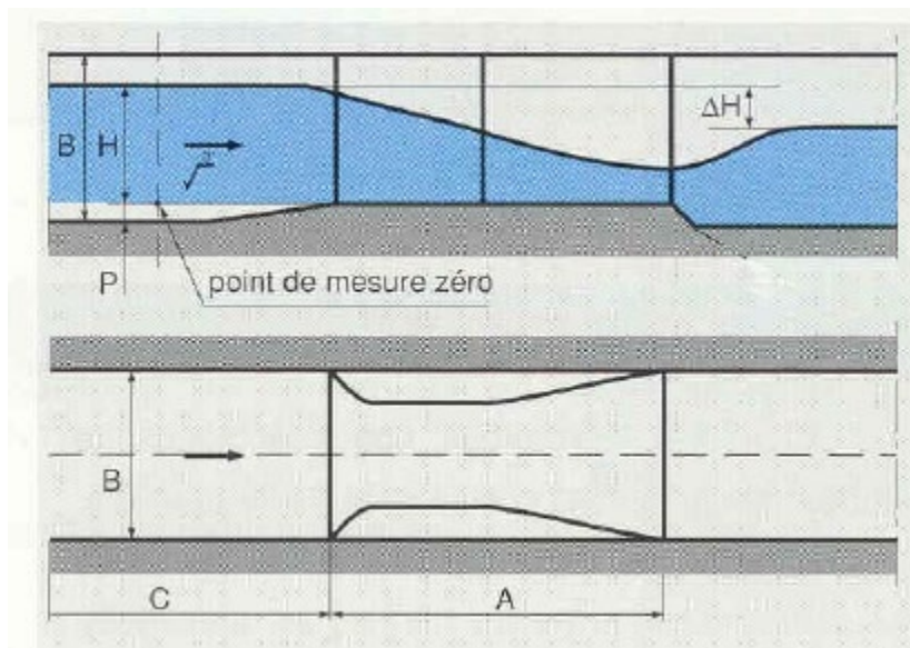
Figuur 10 Schematische voorstelling van meetgoot type Hydrologic serie 1254 met aanduiding van maten (bron: Elscolab ® ) [B: breedte van het aanvoerkanaal; A: lengte van de vernauwing; C: lengte van het aanvoerkanaal P: hoogte van de helling/verhoging]
