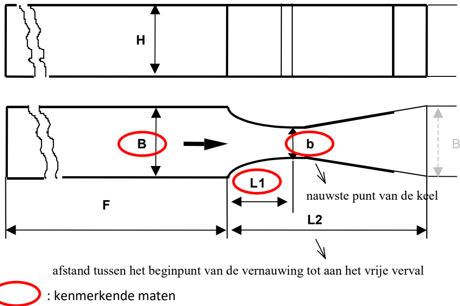
Figuur 7 Schematische voorstelling van Venturi meetgoot type Khafagi QV met aanduiding van maten (bron: VMM) [B: breedte van het aanvoerkanaal; b: breedte van de keel; L1: radius van de boog; L2: lengte afvoerkanaal vanaf de vernauwing/keel; F: lengte aanvoerkanaal-hartlijn meetput; H: hoogte van de meetgoot]
