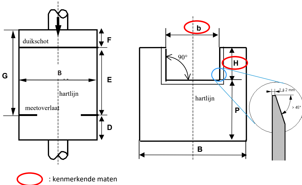
Figuur 13: Schematische voorstelling van meetschot met rechthoekige overlaat met insnoering met aanduiding van maten (bron: VMM) [B: breedte van het aanvoerkanaal/meetput; b: breedte van de rechthoekige uitsnijding; H: hoogte van de rechthoekige uitsnijding; P: hoogte van de onderzijde van de rechthoekige uitsnijding ten opzichte van de vloer; D: stroomafwaartse afstand van het meetschot tot aan de putwand; E: afstand tussen duikschot en meetschot; F: stroomopwaartse afstand van putwand tot aan het duikschot; G: stroomopwaartse afstand van de putwand tot aan het meetschot; H: hoogte van de rechthoekige uitsnijding]
