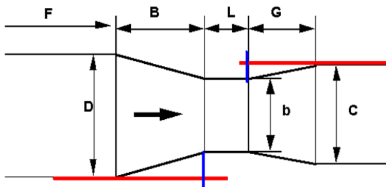
Figuur 12: Opmeting B en G bij type Parshall (bron: VMM)
