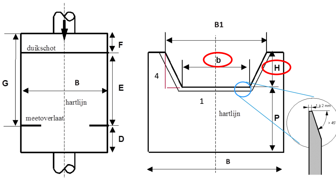
Figuur 14: Schematische voorstelling van meetschot Cipoletti met trapezoidale overlaat met aanduiding van maten (bron: VMM) [B: breedte van de meetput, waarin het meetschot geïnstalleerd werd; B1: breedte van de bovenzijde van de trapeziumvormige uitsnijding; b: breedte van de onderzijde van de trapeziumvormige uitsnijding; H: hoogte van de uitsnijding; P: hoogte van de onderzijde van de rechthoekige uitsnijding ten opzichte van de vloer; D: stroomafwaartse afstand van het meetschot tot aan de putwand; E: afstand tussen duikschot en meetschot; F: stroomopwaartse afstand van putwand tot aan het duikschot; G: stroomopwaartse afstand van de putwand tot aan het meetschot; H: hoogte van de rechthoekige uitsnijding]
