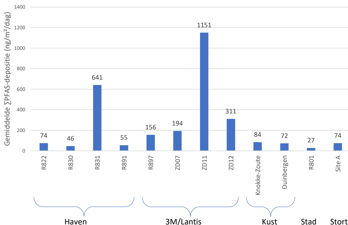
Figuur 29: Gemiddelde ΣPFAS depositie op de verschillende meetlocaties (Antwerpse Haven, 3M/Lantis, Kust, Stedelijke achtergrond en Stortplaats).
