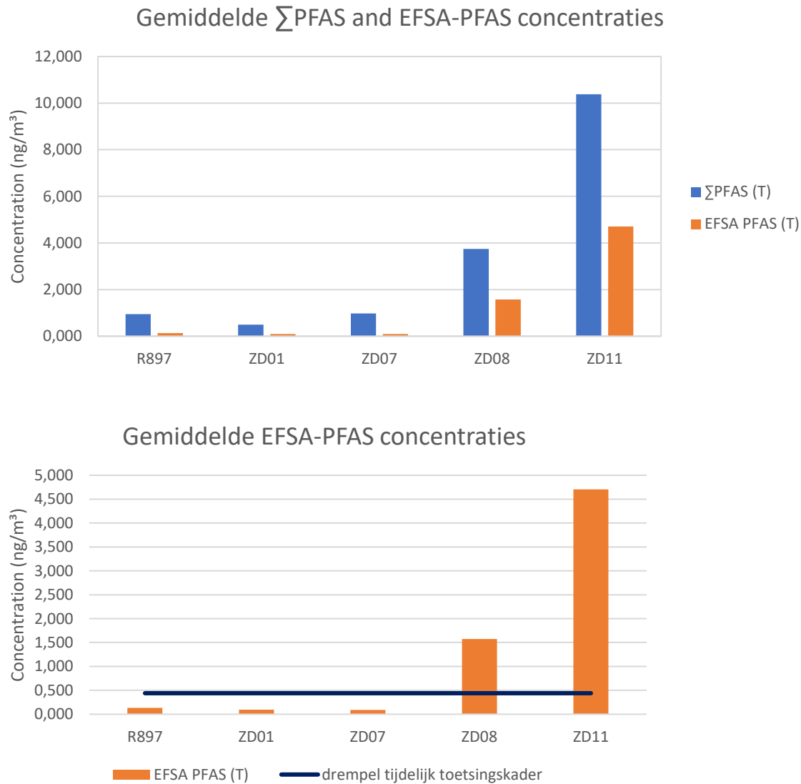
Figuur 15: Gemiddelde \Sigma PFAS en EFSA-PFAS concentratie op meetlocaties in de omgeving van 3M gedurende de meetperiode (boven). De EFSA-PFAS concentraties liggen op twee meetlocaties boven de toetsingswaarde van 0,44 ng/m 3 (onder).
