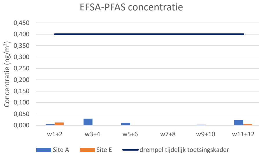
Figuur 12: EFSA-PFAS concentraties in de buurt van de stortplaats. De concentraties liggen ver beneden de toetsingswaarde.
