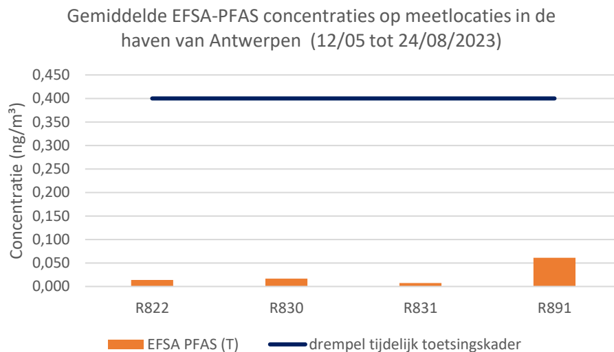
Figuur 19: Gemiddelde \Sigma PFAS(T) en EFSA-PFAS(T) concentratie op meetlocaties in de haven gedurende de meetperiode (boven). De EFSA-PFAS concentraties liggen op elke meetlocatie onder de toetsingswaarde van 0,4 ng/m 3 (onder).
