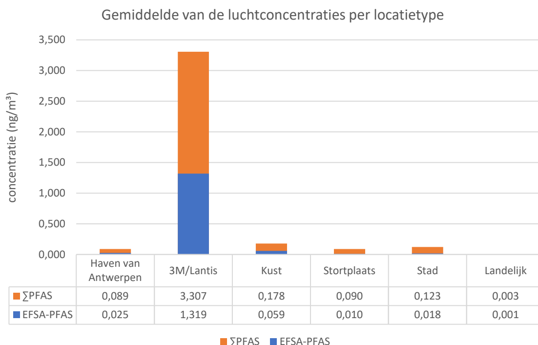
Figuur 22: Gemiddelde van de luchtconcentraties van \Sigma PFAS en EFSA-PFAS op de verschillende type locaties.
